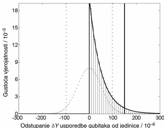
Slika 11.: Rezultati za model usporedbe gubitka umjeravanja mjerila snage u slučaju x_1 = x_2 = 0 , s u(x_1) = u(x_2) = 0,005 i r(x_1, x_2) = 0 (podtočke 9.4.2.2.2, 9.4.2.2.6, 9.4.2.2.9 i 9.4.2.2.11)
