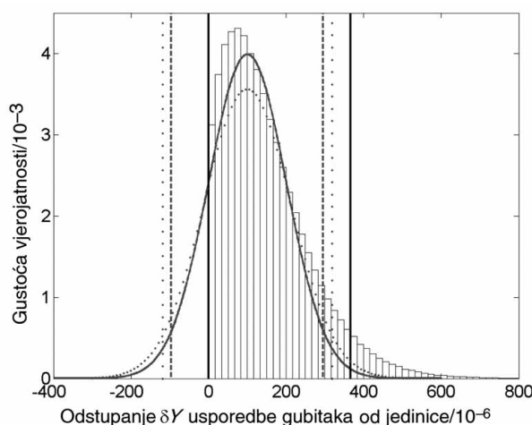
Slika 13.: Kao slika 11. osim što je x_1 = 0,010 , a funkcija gustoće vjerojatnosti koja nastaje iz okvira nesigurnosti GUM-a s članovima prvog reda (krivulja s višom vršnom vrijednošću) i višeg reda (krivulja s nižom vršnom vrijednošću) (podtočke 9.4.2.3.1, 9.4.2.3.3, 9.4.2.4.1 i 9.4.3.3)
