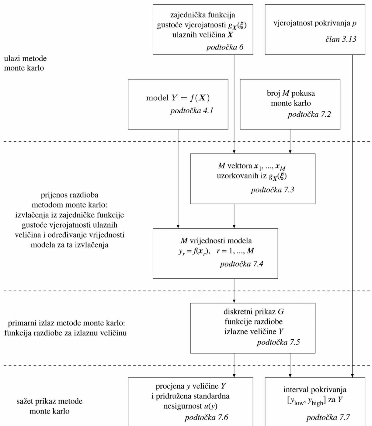
Slika 4.: Faza prijenosa i prikaza u sažetu obliku određivanja vrijednosti nesigurnosti uporabom metode monte karlo (MCM) za primjenu prijenosa razdioba (podtočke 5.9.6 i 7.1)
