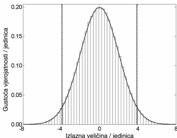
Slika 6.: Aproksimacija funkcije gustoće vjerojatnosti veličine Y za model (21) dana a) okvirom nesigurnosti GUM-a i b) metodom monte karlo (podtočke 9.2.2.6 i 9.2.3.3), pri čemu je svakoj ulaznoj veličini X_i dodijeljena standardna Gaussova funkcija gustoće vjerojatnosti. "Jedinica" označuje bilo koju jedinicu
