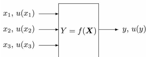
Slika 3.: Ilustracija zakona prijenosa nesigurnosti za N = 3 neovisne ulazne veličine (podtočke 5.4.4 i 5.6.3).
